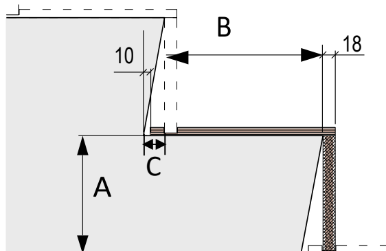
Contremarches inclinés
