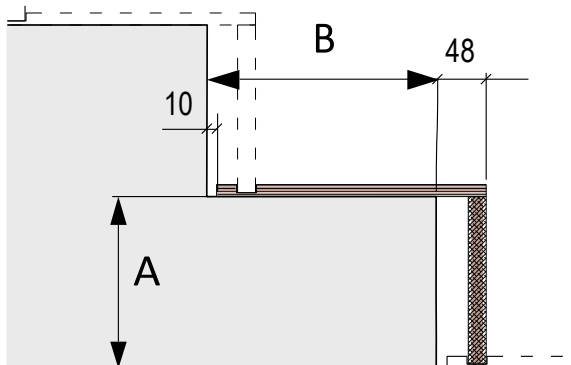
Contremarches droites
