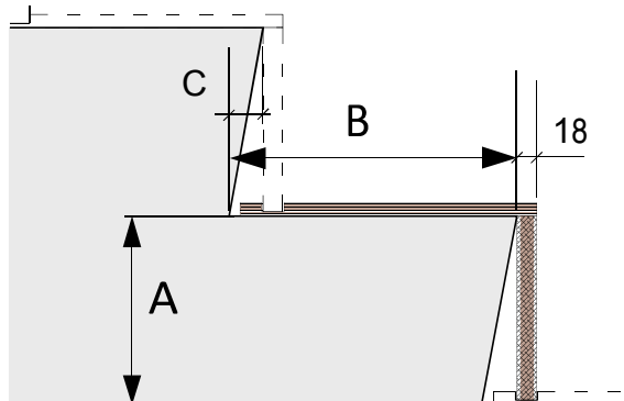
Contremarches inclinés ou nez de marche
